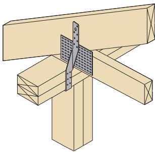
LTS, MTS & HTS
